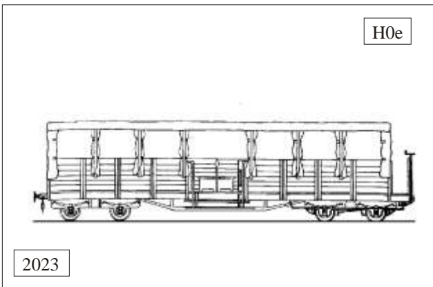
Sommerwagen Trusetalbahn
